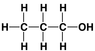
1-propanol
