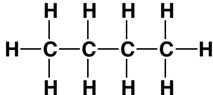
butane
