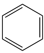
benzene
